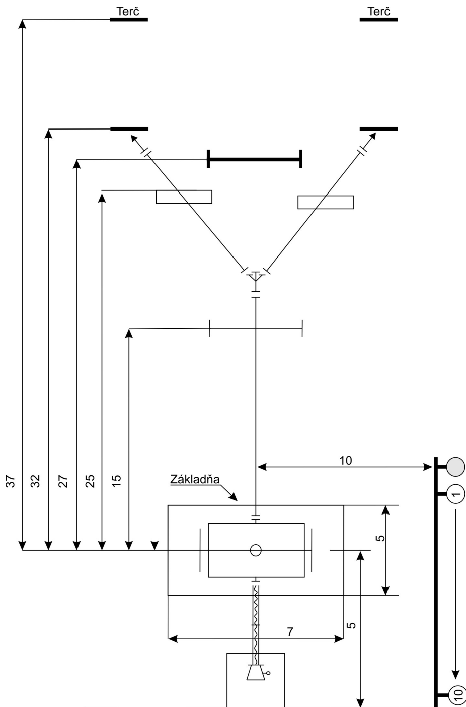
Nákres vykonania požiarneho útoku
